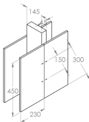
Illustration 3 : Dimensions de l'éprouvette en mm, agrafes orientées à 90°
