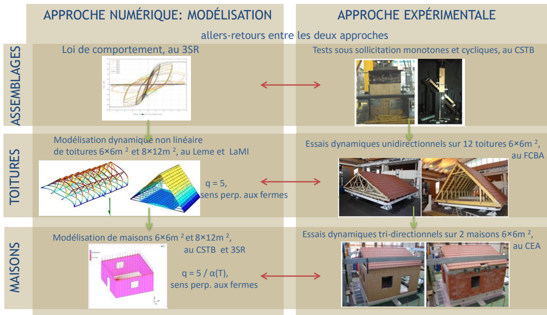
Illustration 8 : Démarche scientifique développée dans SISBAT basée sur une approche multi-échelles et sur le couplage éléments finis stochastiques / expérimentation
