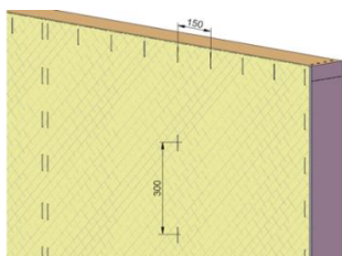
Illustration 4 : Positionnement des agrafes dans les murs
