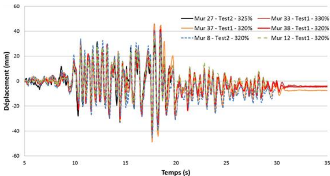
Illustration 6 : Signaux temporels en déplacement en tête des murs pointés N°8 et 12 (courbes en pointillés) et des murs agrafés N° 27, 33, 37 et 38 (courbes pleines), pour le séisme 1 à 1 g
