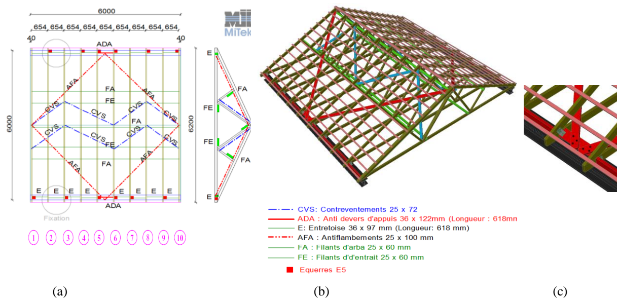
Illustrations 7 : Description des toitures en dimensions 6×6 m 2 pour les essais sur table vibrante (source MiTek)
